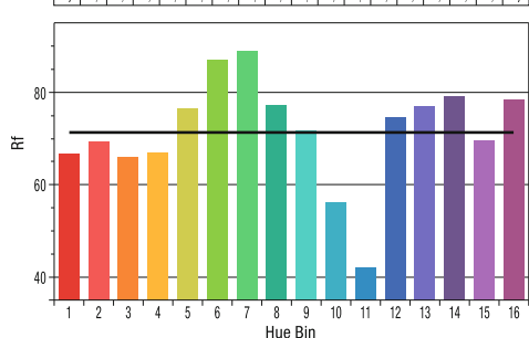
FARBWIEDERGABE – TM-30-15
