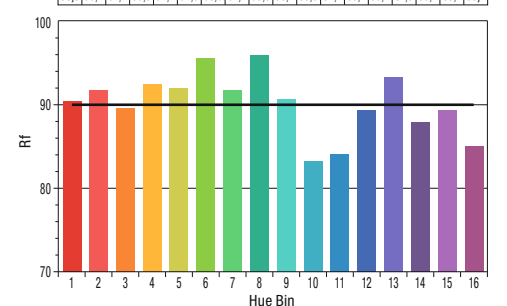
FARBWIEDERGABE – TM-30-15
