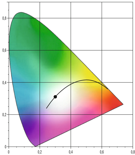
FARBWIEDERGABE – CRI
