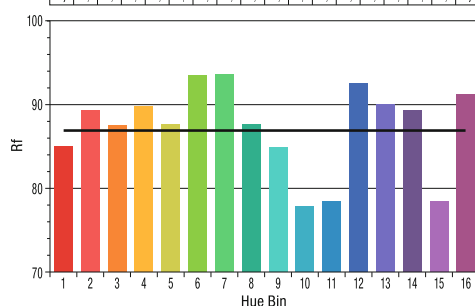
FARBWIEDERGABE – TM-30-15
