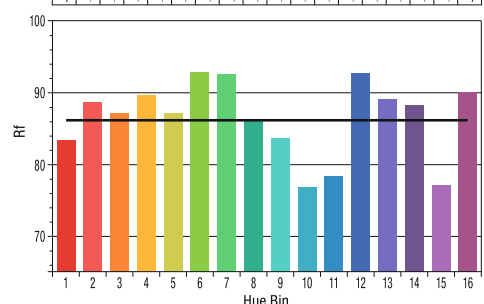
FARBWIEDERGABE – TM-30-15
